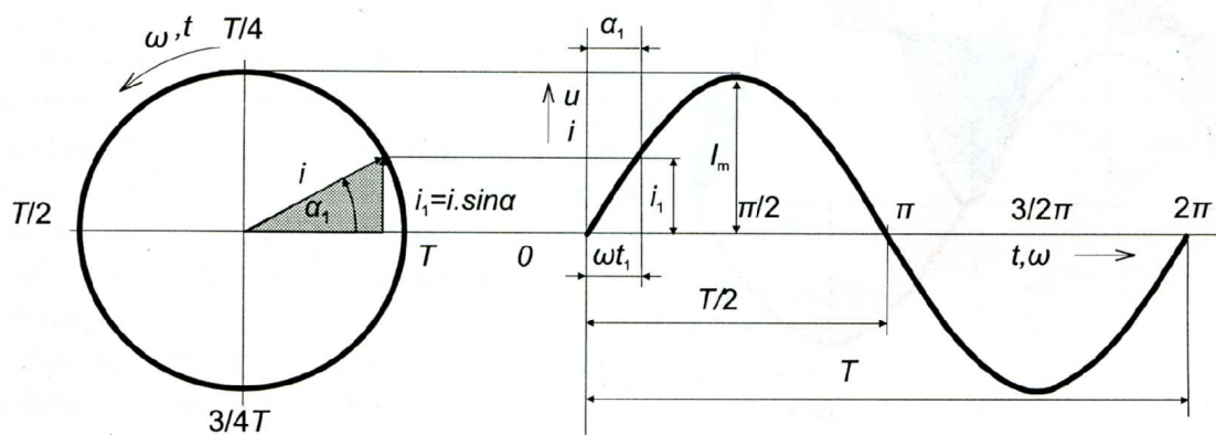
Obr. 61. Časový průběh sinusových veličin
